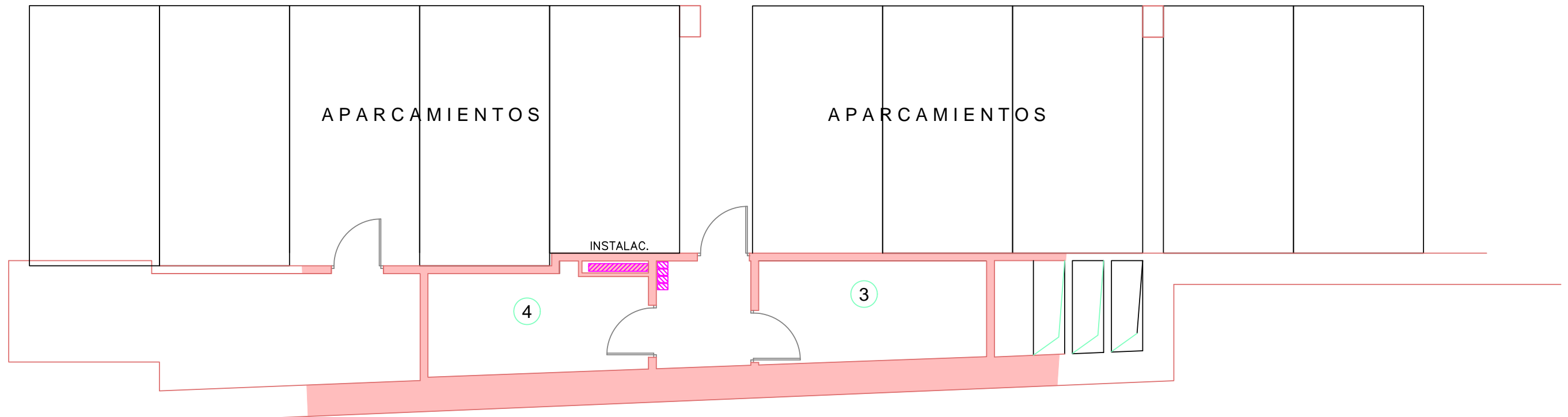
TRASTEROS ESTADO REFORMADO SOTANO 3º Escala 1/100
